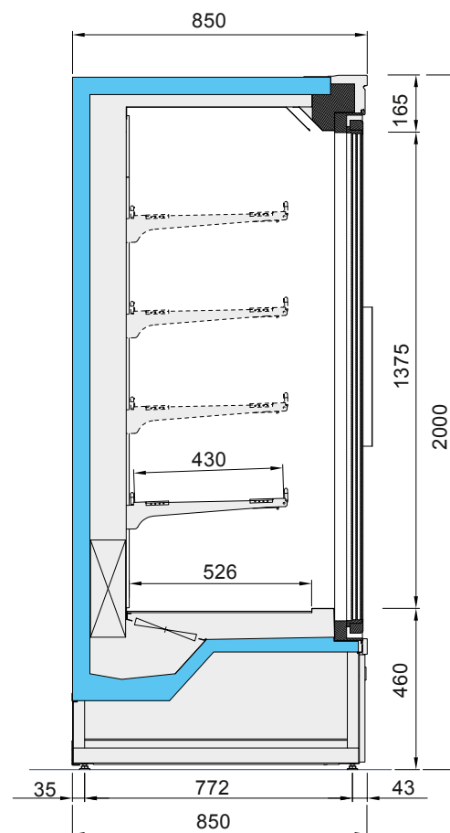
ONYX BT: P 850 H 2000
